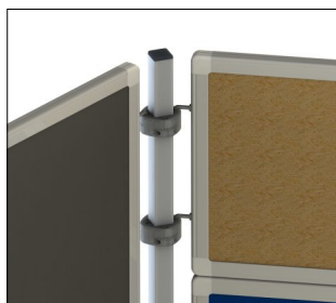
Detail uchycení tabulí na stojnu pomocí závěsných háčků
