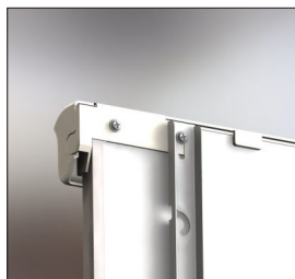
Detail sklopené boční lišty pro zavěšení papíru
