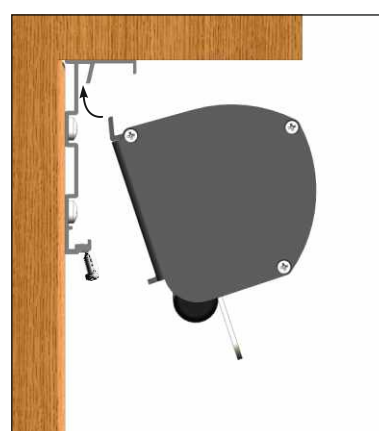
BOČNÍ POHLED
